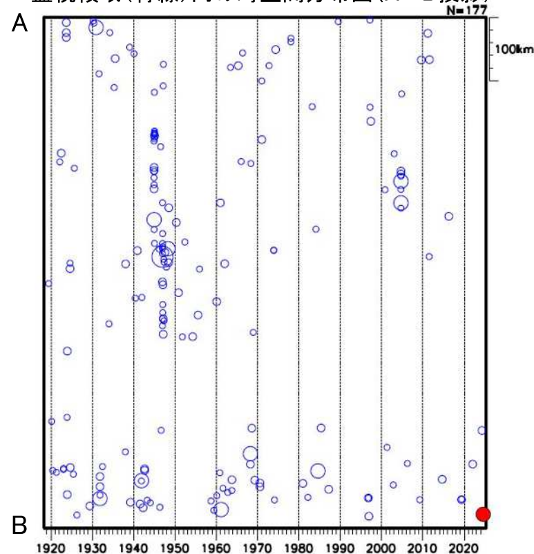
監視領域(青線)内の地震活動経過図
