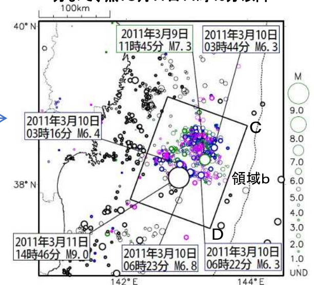
震央分布図 (2011年3月9日～3月11日、深さ全て、M全て) 緑: 3月9日、青: 3月10日、桃: 3月11日14時45分まで、黒: 3月11日14時46分以降
