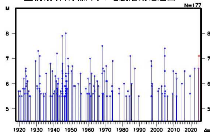
監視領域(青線)内の地震活動経過図
