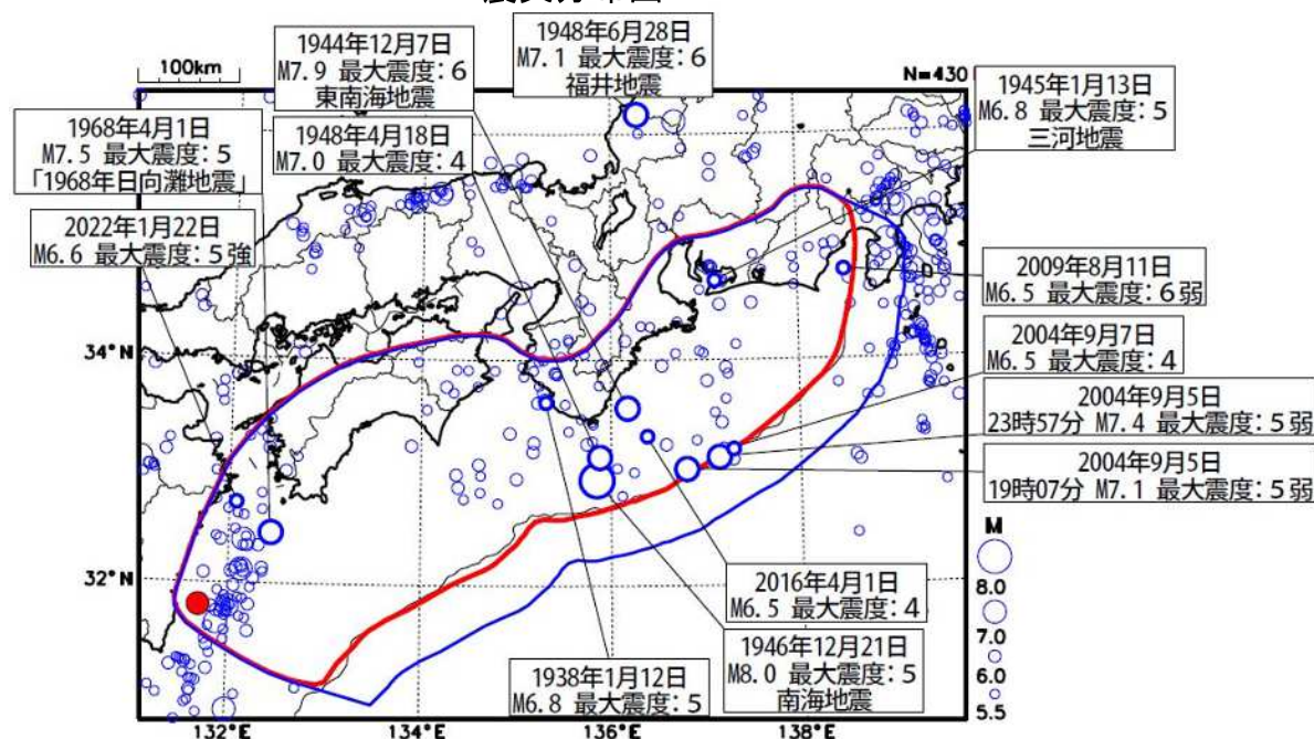
震央分布図
