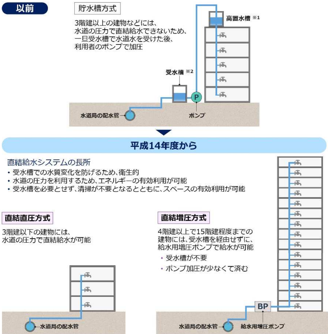
図 3-2-3 直結給水システム
