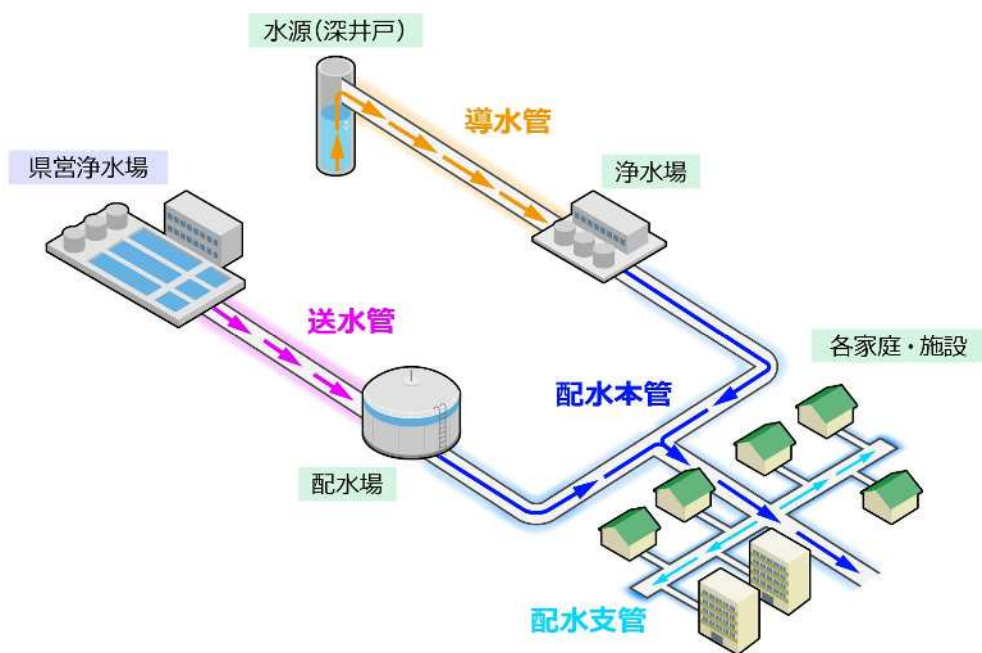
図 2-2-3 管路の構成図
