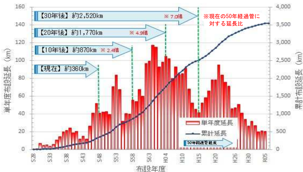
さいたま市の下水道管渠布設延長（令和5年度末）
