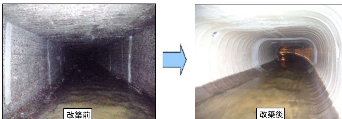
老朽化対策（管きょ更生工法）[大門浅間2号幹線]
