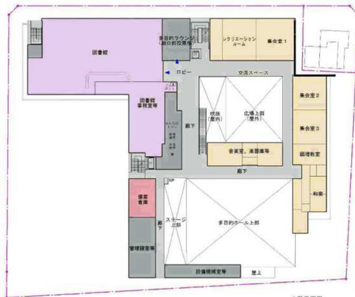
2階平面図
