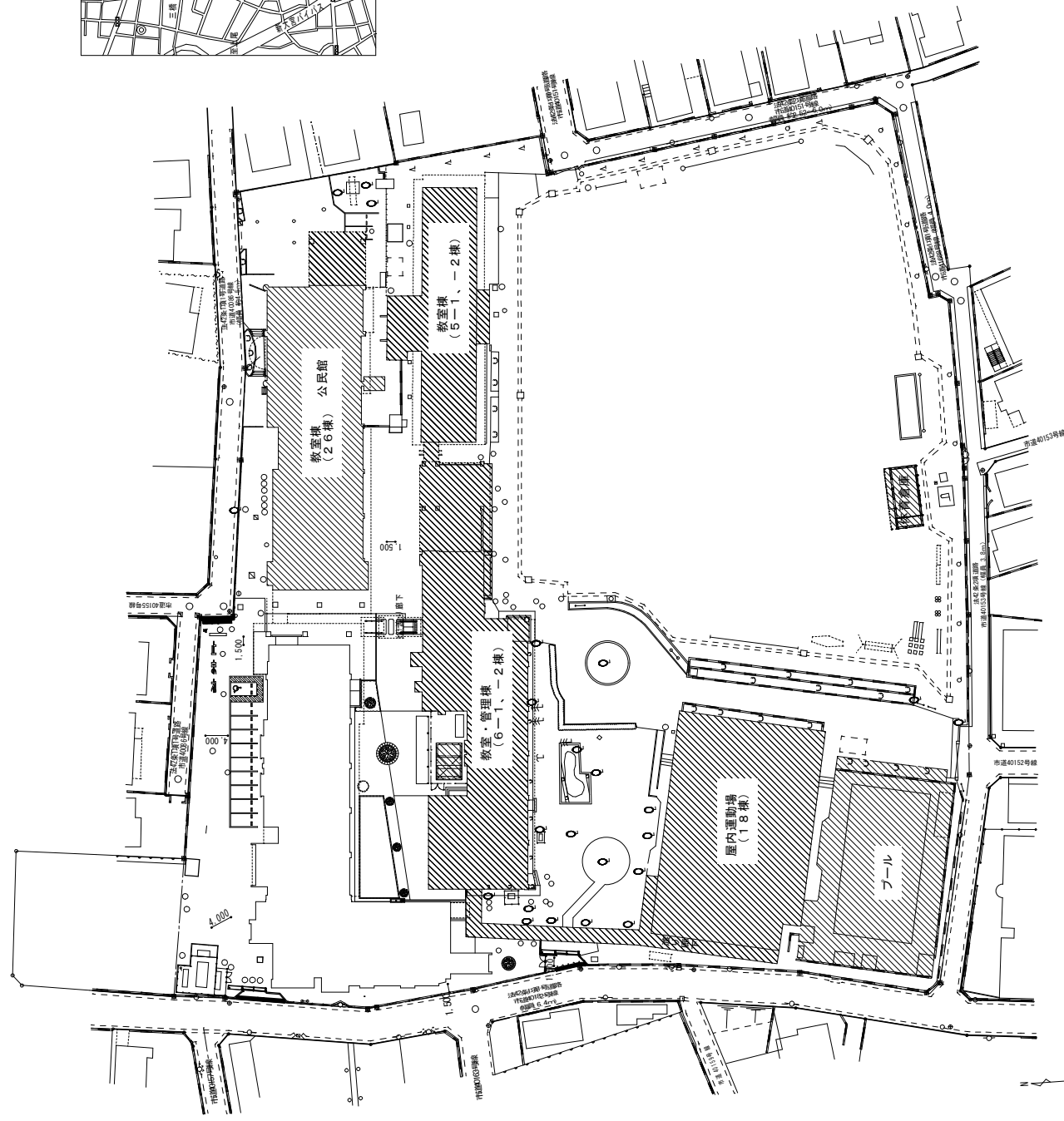
配置図
