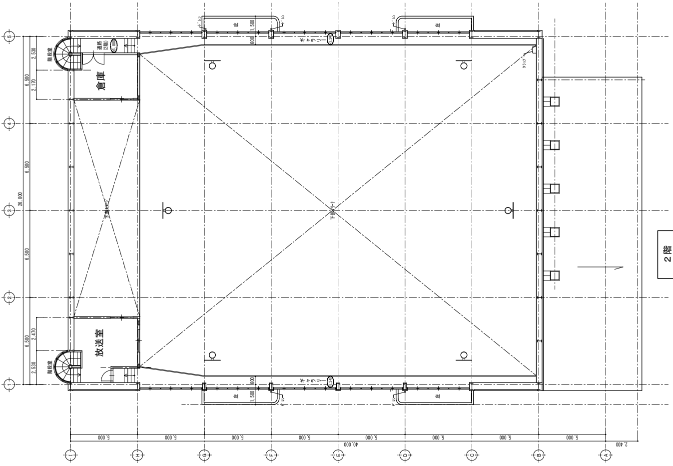
屋内運動場 (18棟) 平面図
