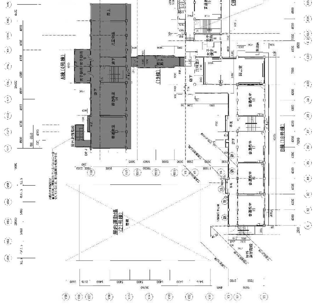
3階平面図
