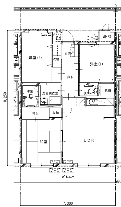
3LDK平面図
