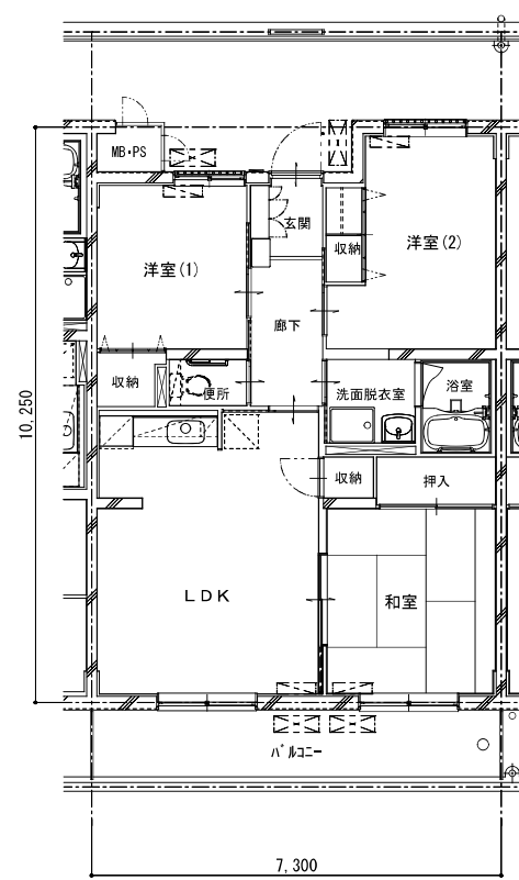
3LDK平面図
