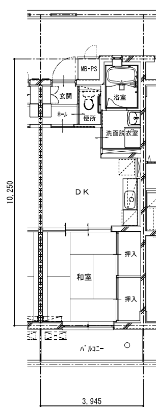
1DK平面図
