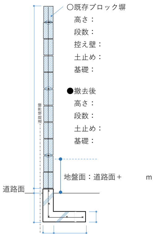
断面図
