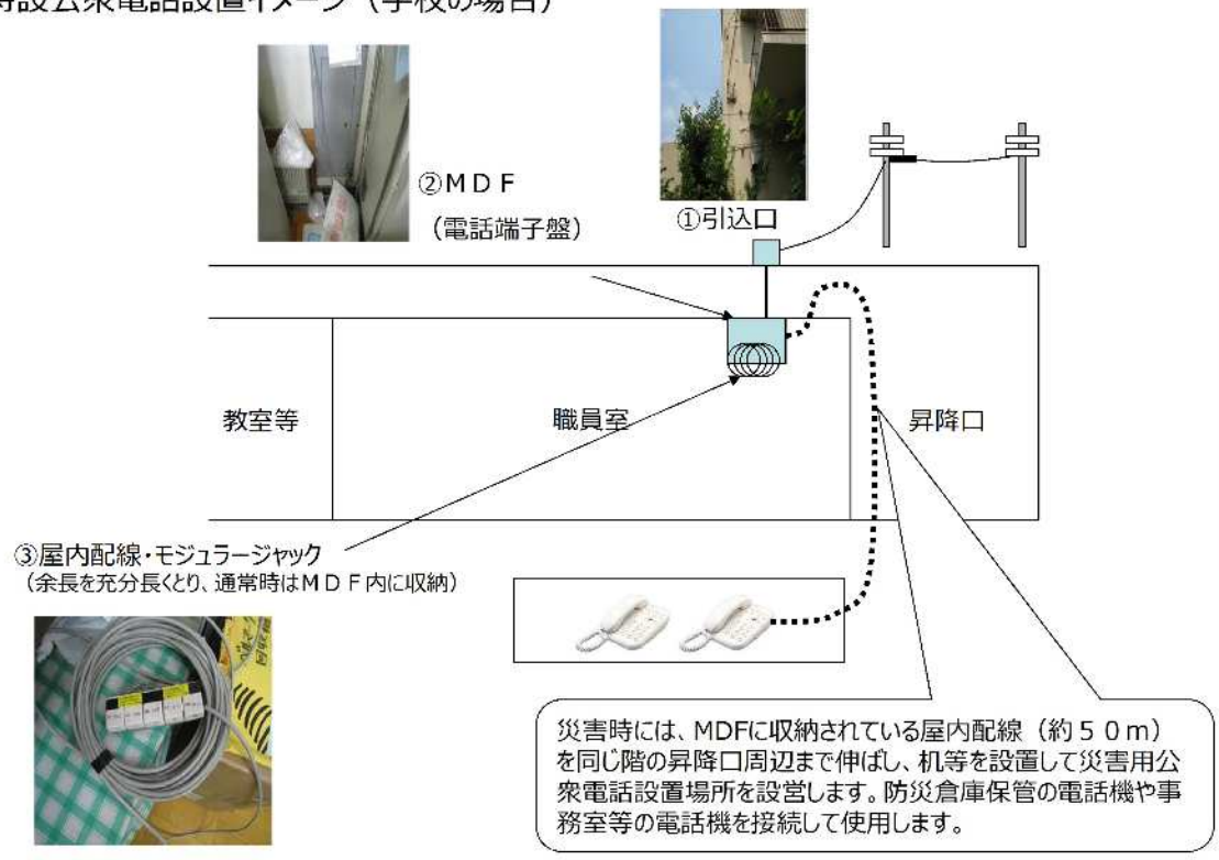
特設公衆電話設置イメージ（学校の場合）
