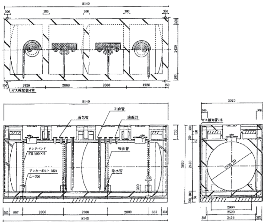
30KL 中仕切 15 : 15 (直径 2.4 m)
