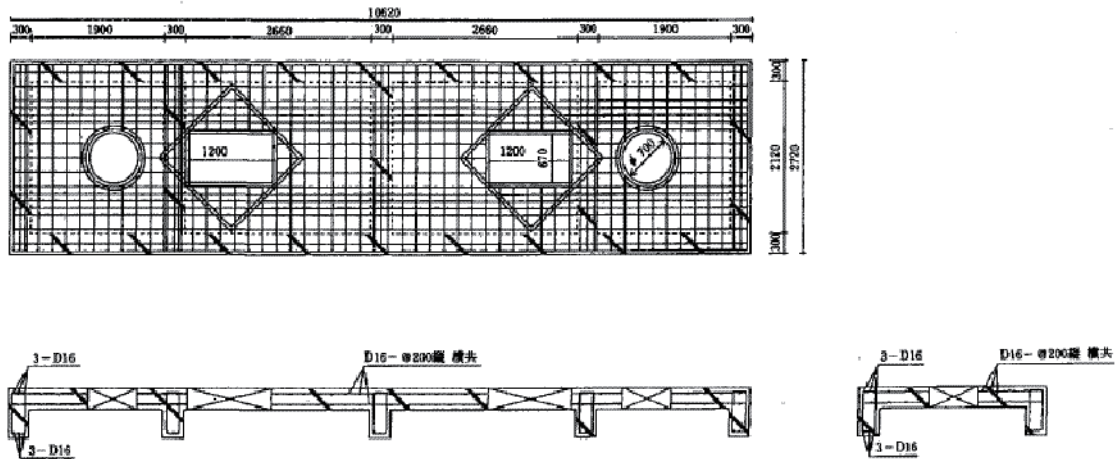
図4-25-2-2 コンクリート被覆タンク配筋図
