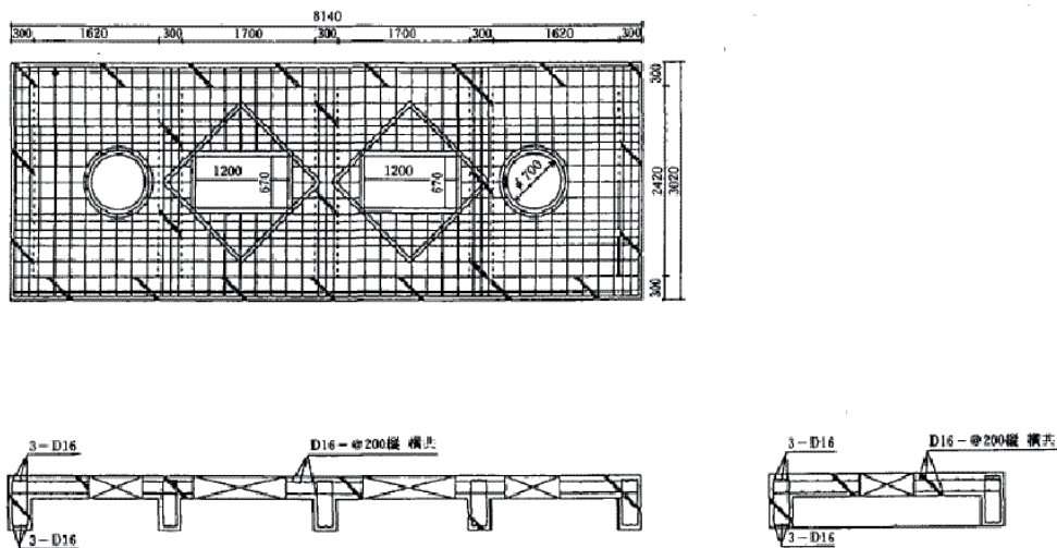
図4-25-1-2 コンクリート被覆タンク配筋図
