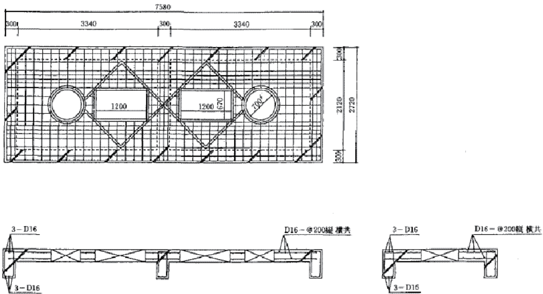
図4-25-4-2 コンクリート被覆タンク配筋図
