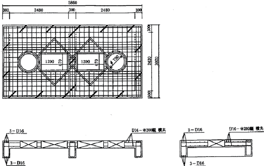
図4-25-3-2 コンクリート被覆タンク配筋図
