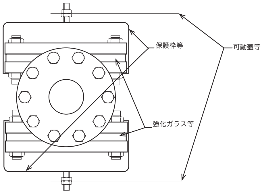
A-A 矢視図
