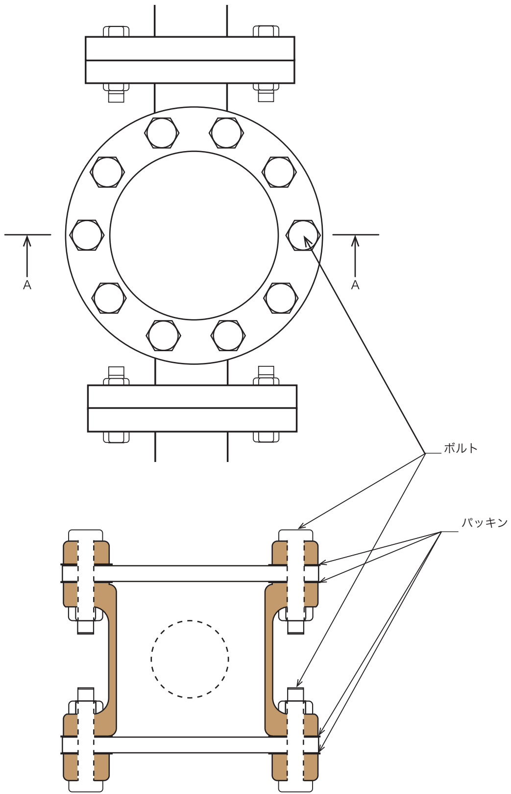
A-A断面図
