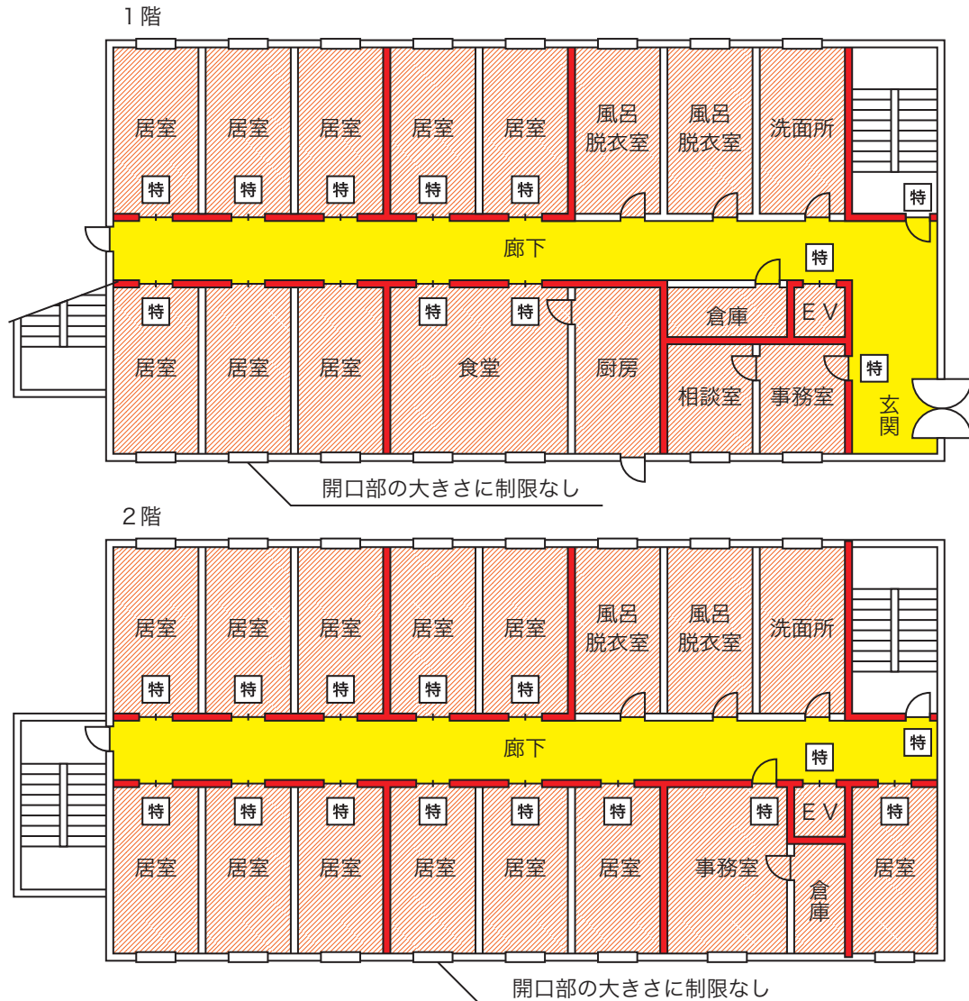
別図3 省令第12条の2第1項第2号
