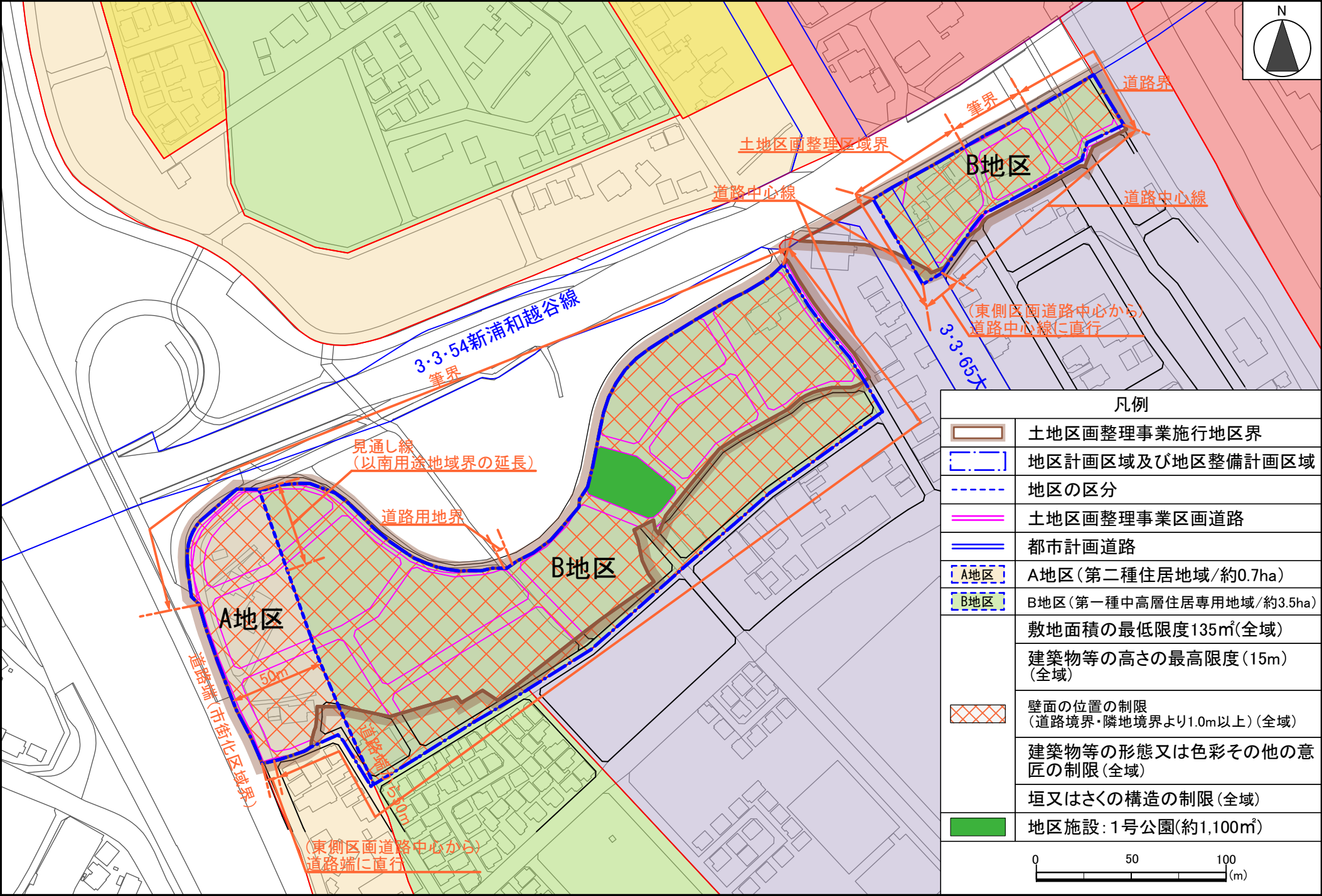
地区整備計画図 大門下野田地区
