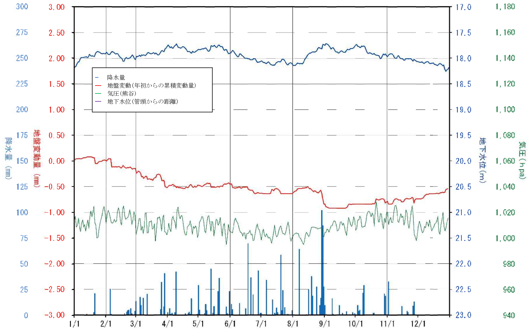
図-2.1.3 岩槻観測所 地盤変動・地下水位変動図
