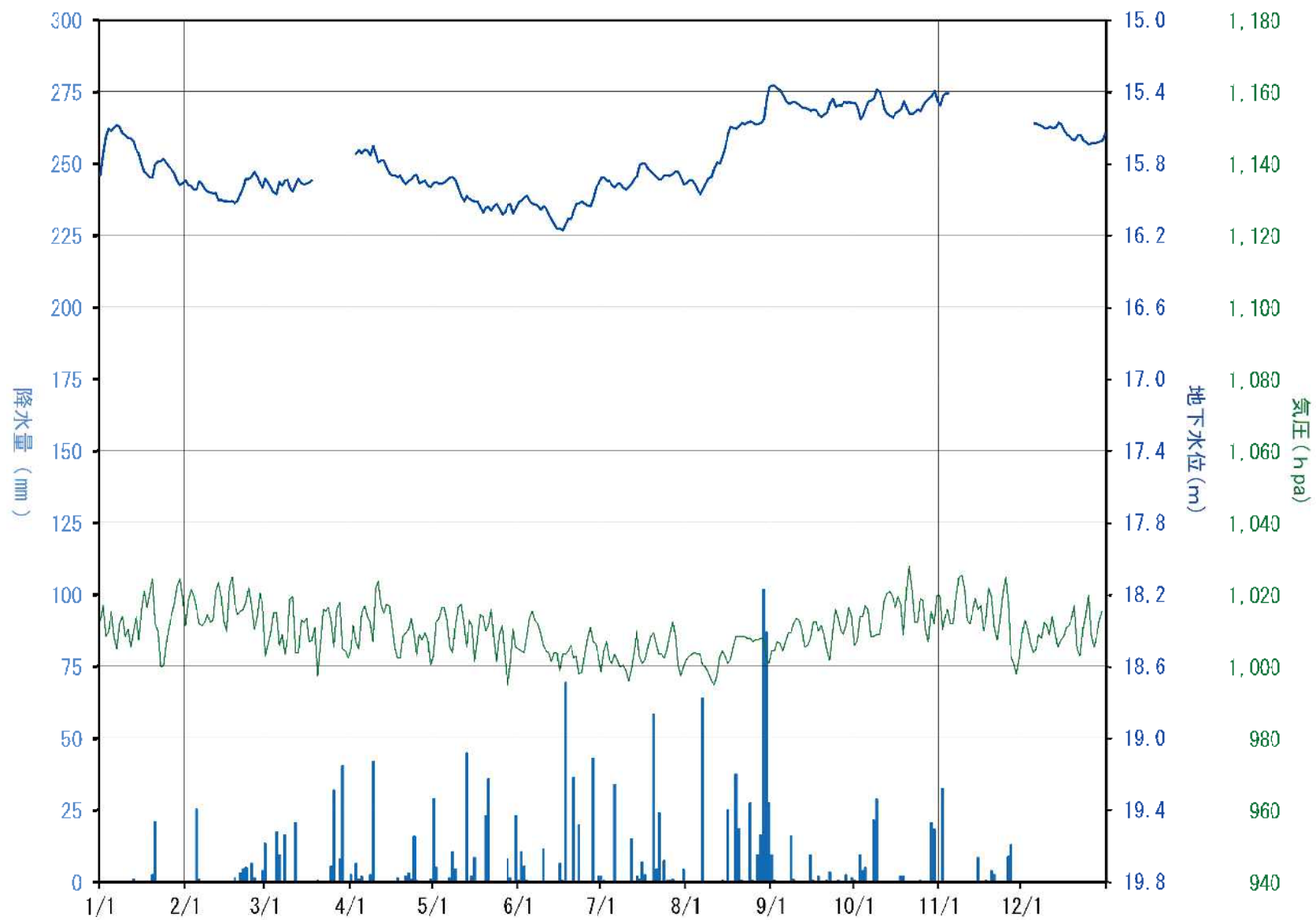
図-2.1.2 浦和東観測所 地下水位変動図
