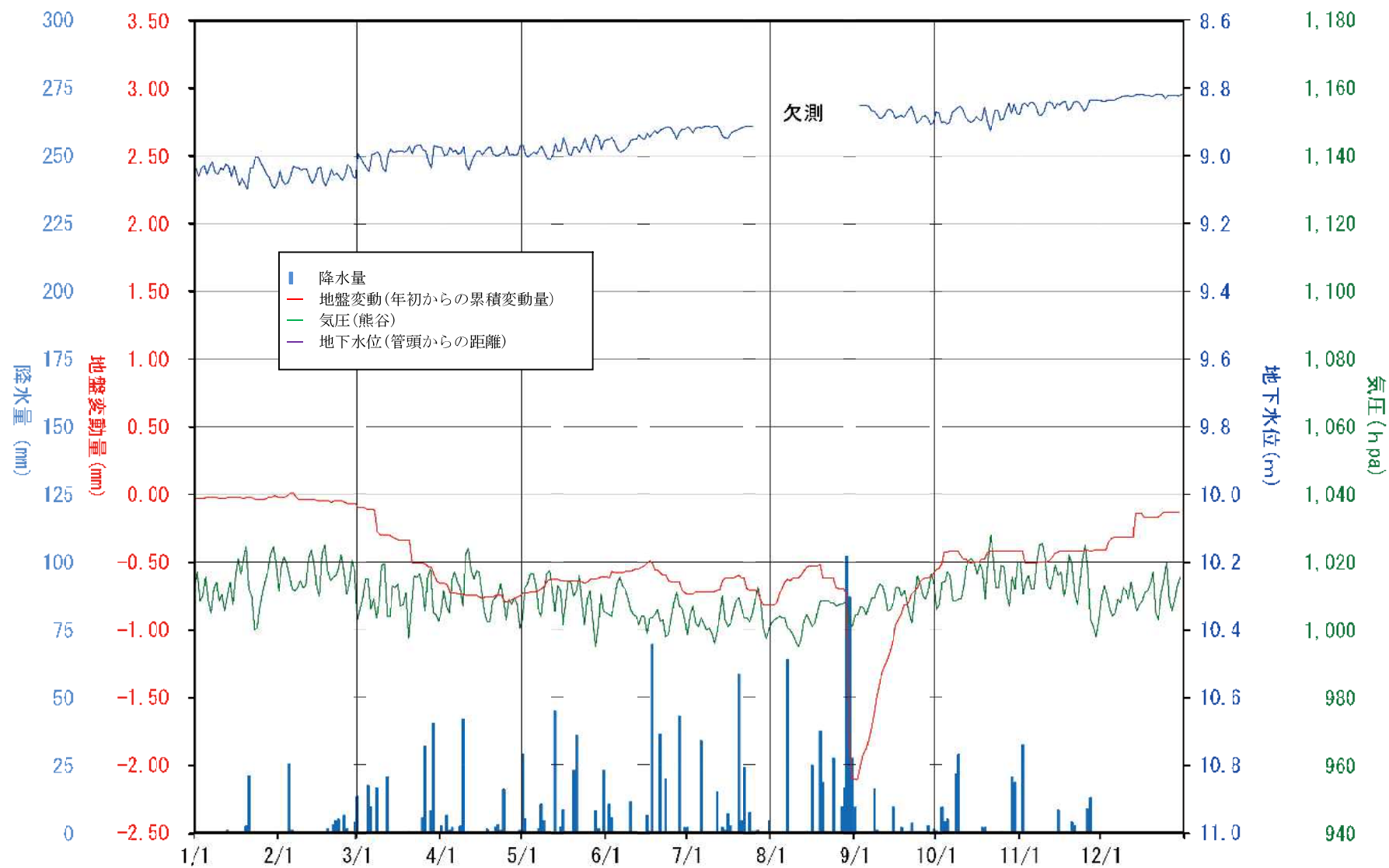
図-2.1.1 大宮観測所 地盤変動・地下水位変動図
