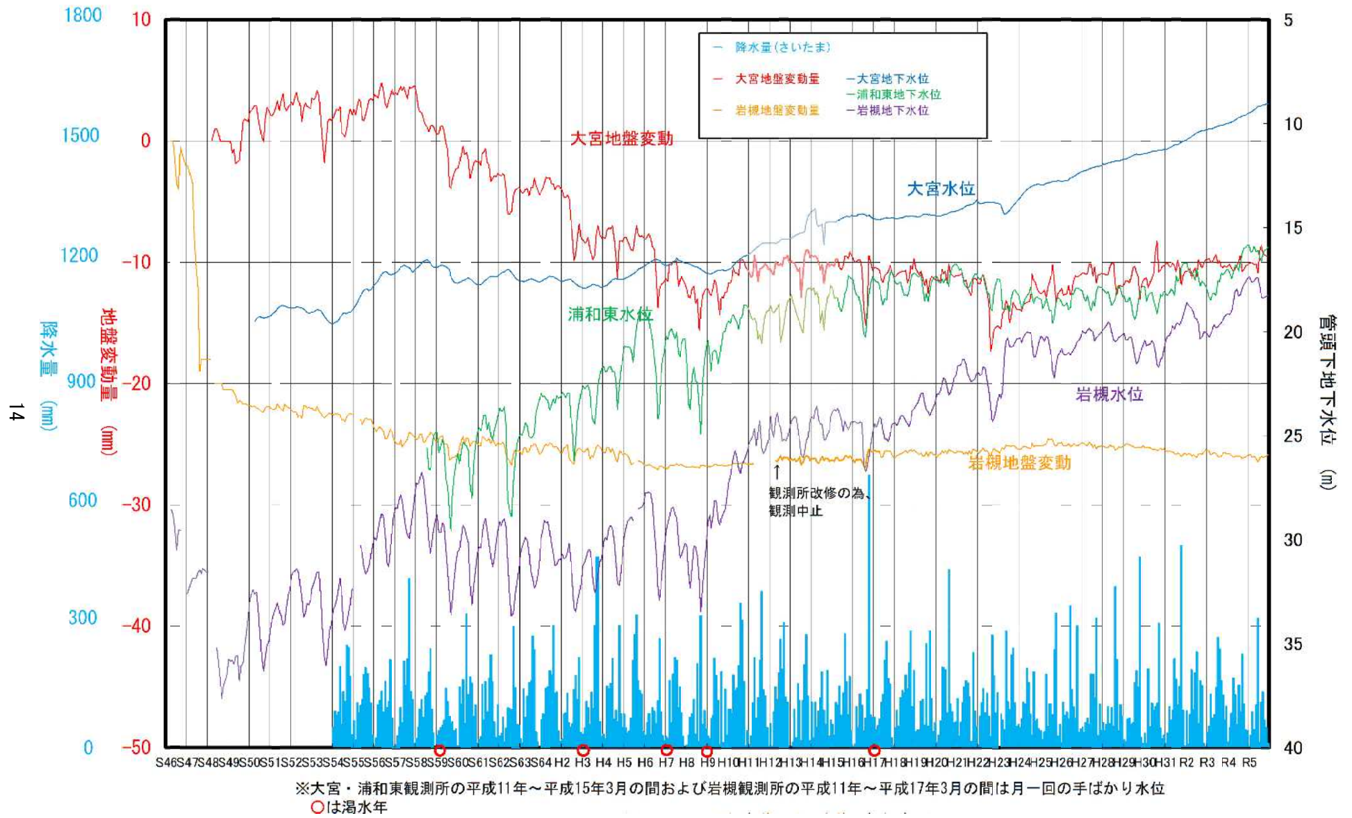
図-2.3.1 地盤沈下・地下水水位 経年年化図
