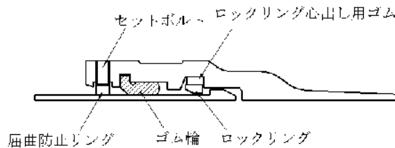
図 4-10 NS形異形管（呼び径 75～250）の継手の接合
